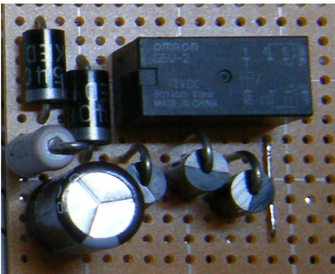
切替用ル-とダイオード・コンデンサ・抵抗
